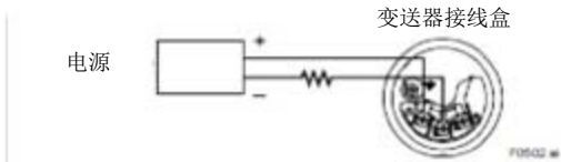
图 5.2 电源连接
