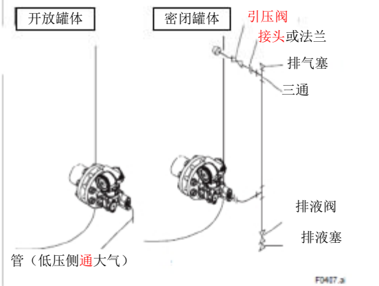
图 4.7 配管示例（EJ□210□）
