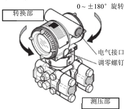
图 3.12 旋转转换部（左侧高压型）
