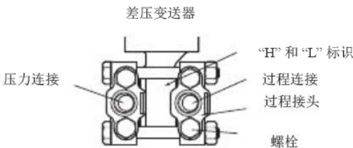
图 4.1 膜盒上的“H”和“L”标识
