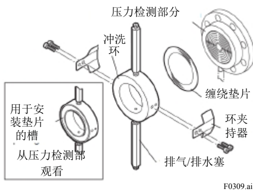
图 3.9 安装到压力检测部
