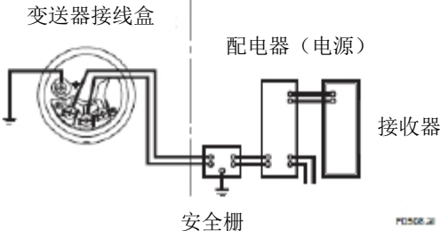
图 5.8 变送器与配电器连接
