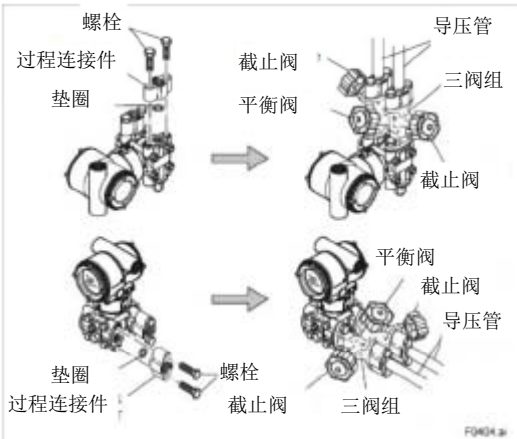
图 4.4 三阀组（直接安装型）
