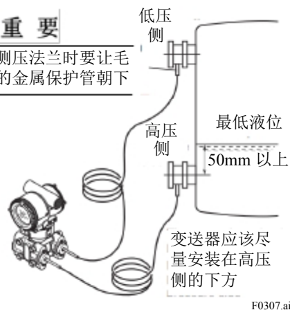
图 3.7 液灌隔膜密封安装
