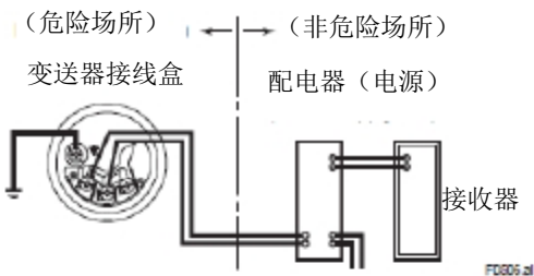
图 5.6 变送器与配电器连接
