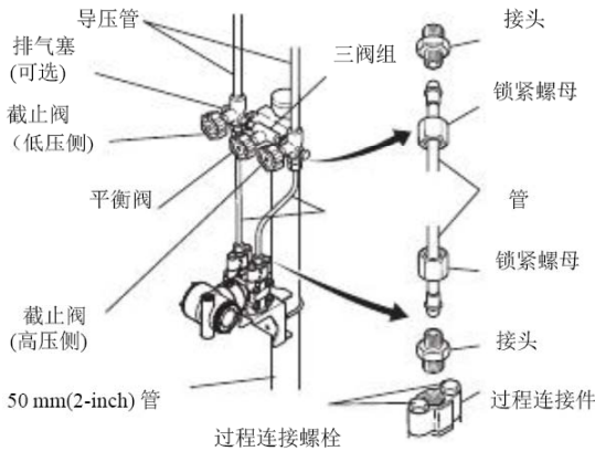
图 4.3 三阀组（配管型）
