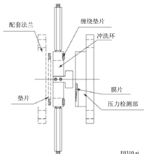
图 3.10 安装到过程法兰
