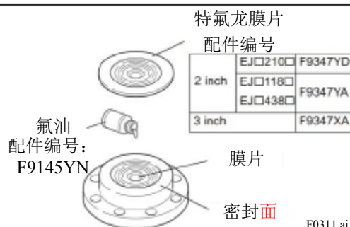
图 3.11 特氟龙膜片 粘贴
