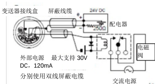
图 5.4 状态输出连接
