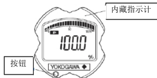
图 6.4 量程设定开关（按钮）
