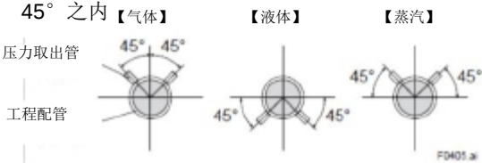
图 4.5 引压阀角度（水平安装）
