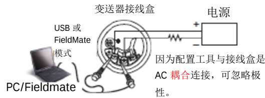
图 5.3 配置工具连接
