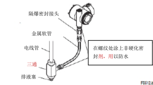
图 5.11 典型隔爆密封接头配线
