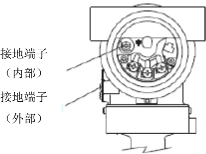
图 5.14 接地端子
