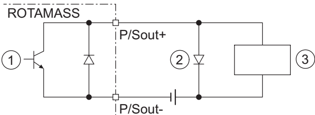
图 38: 配备机电计数器的无源脉冲输出 P/Sout 连接
