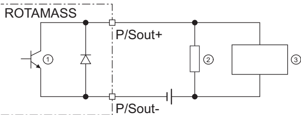
图 37: 配备电子计数器的无源脉冲输出 P/Sout 连接
