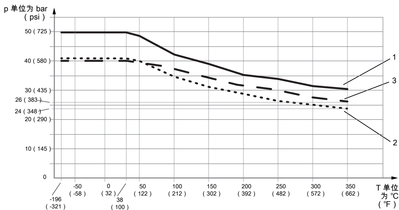
图 9: 与过程介质温度相关的允许过程压力
