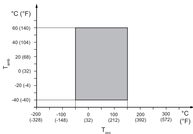
图 17: 允许的过程介质温度和环境温度，一体型（HS4 和 HS8 过程连接形式除外）
