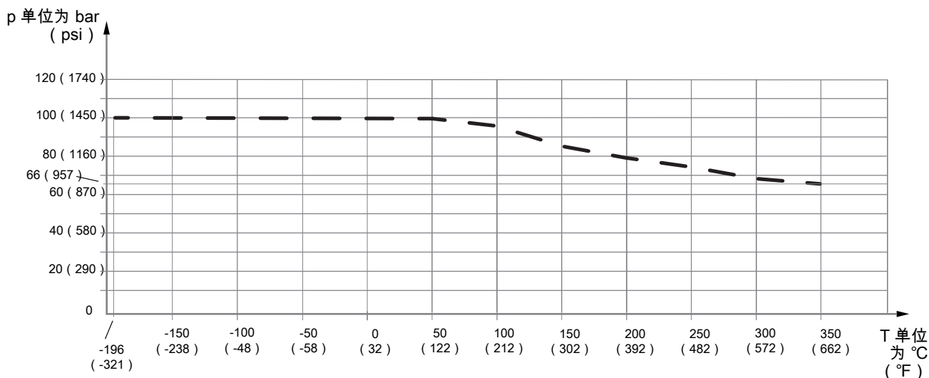
图 11: 与过程介质温度相关的允许过程压力, 符合法兰 EN 1092-1 PN100
