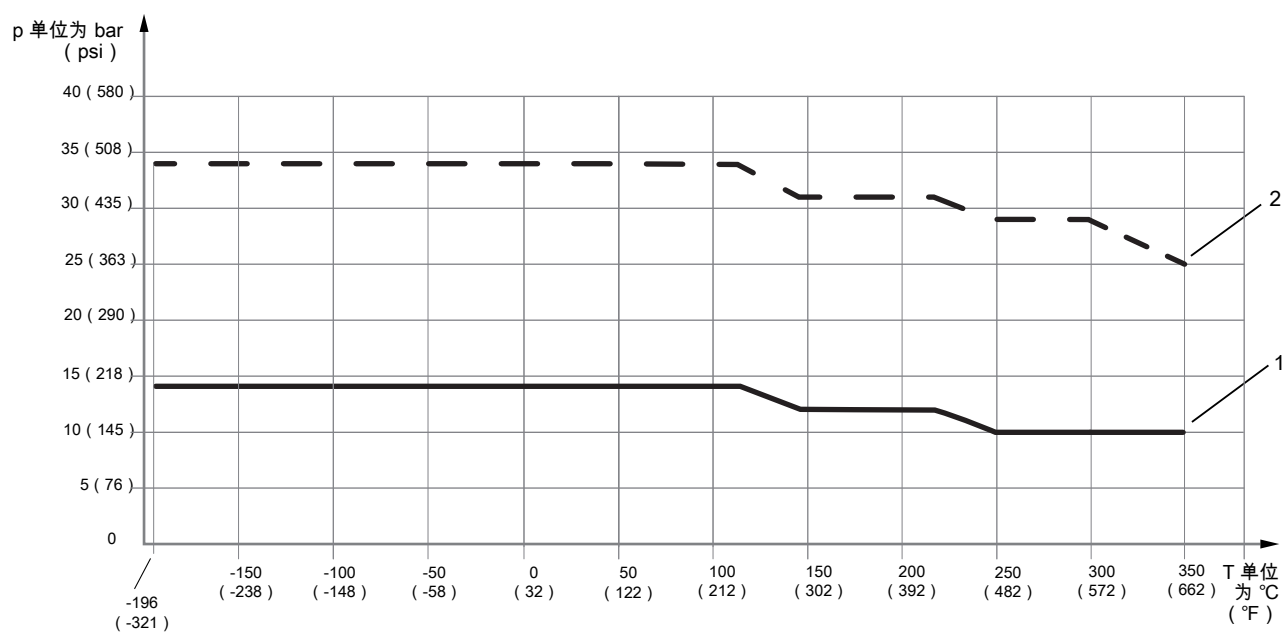
图 12: 与过程介质温度相关的允许过程压力
