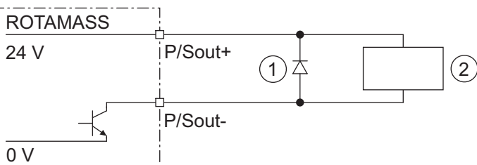
图 35: 配备机电计数器的有源脉冲输出 P/Sout 连接
