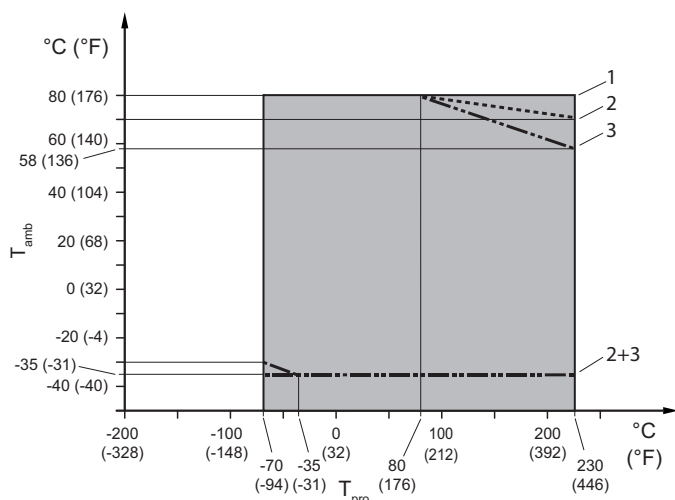
图 22: 允许的过程介质温度和环境温度，分离型
