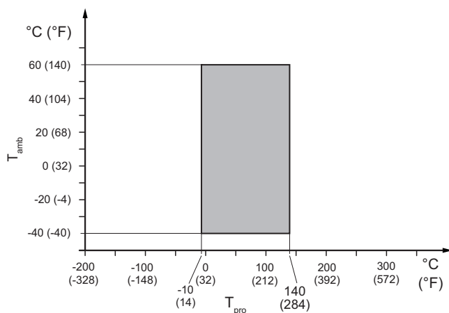
图 18: 允许的过程介质温度和环境温度，一体型，适用于 HS4 和 HS8 过程连接形式
