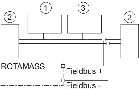
图 46: FOUNDATION 现场总线连接
