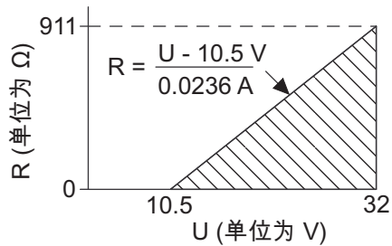
图 30: 最大负载电阻（根据外部供电电源电压）
