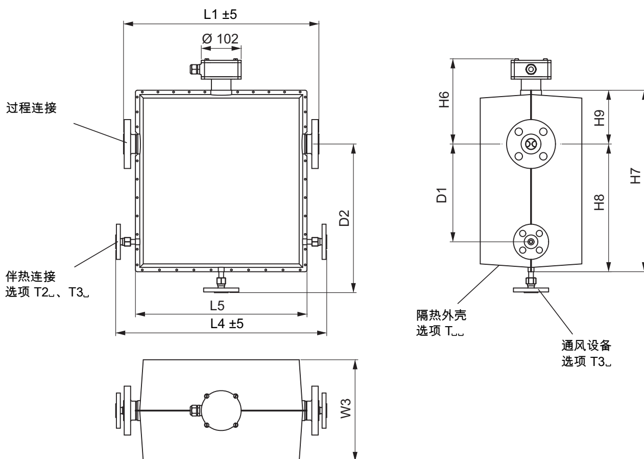
图 26: 尺寸 (毫米): 带隔热外壳的版本, 仅适用于 Intense 34、36 和 38 仪表尺寸
