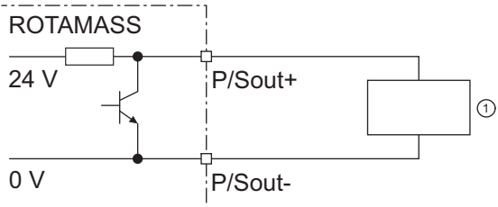
图 40: 配备内部上拉电阻的有源状态输出 P/Sout
