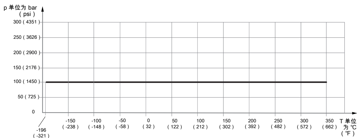
图 16: 与过程介质温度相关的允许过程压力
