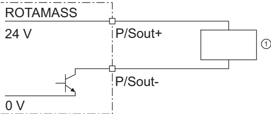
图 39: 有源状态输出连接 P/Sout
