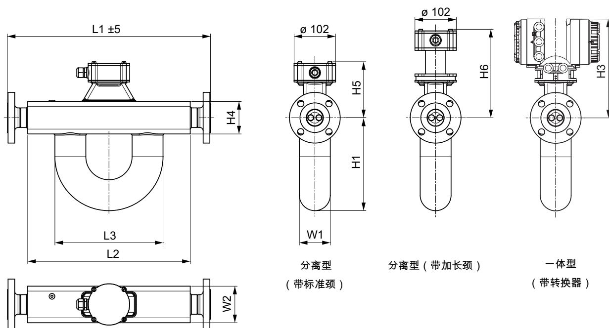
图 25: 尺寸 (毫米)
