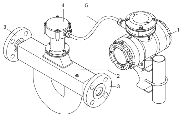
图 4: Rotamass 分离型流量计的配置 - 加长颈
