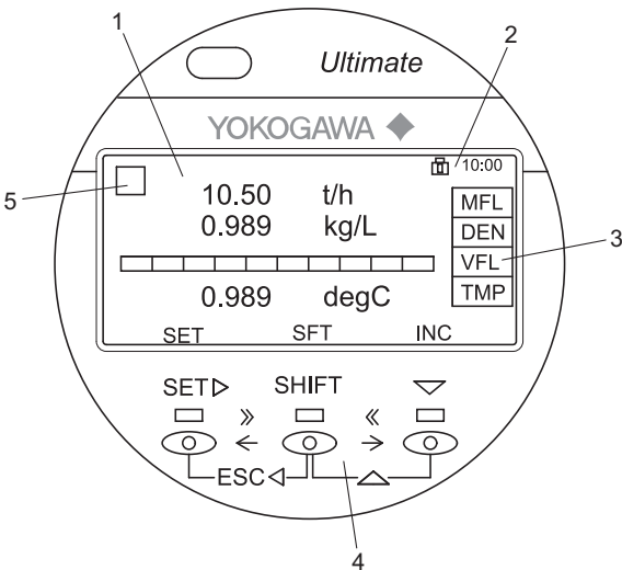
图 47: 显示器布局
