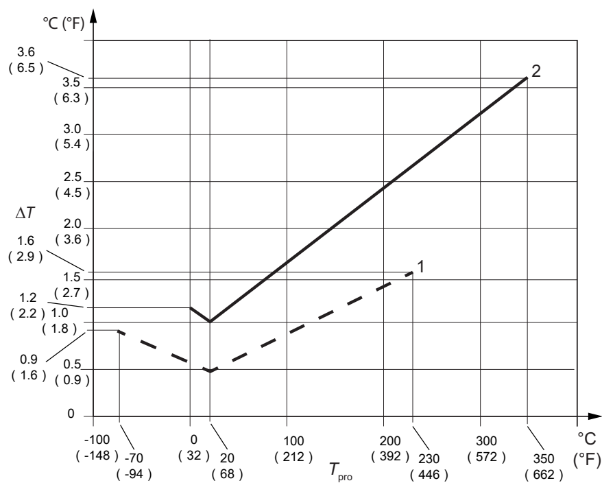
图 6: 温度精度
