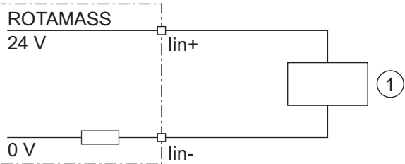
图 32: 外部设备与无源电流输出的连接
