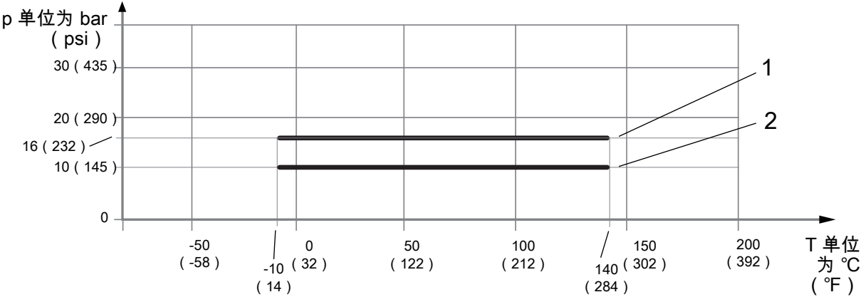
图 13: 与过程介质温度相关的允许过程压力
