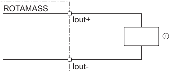
图 29: 有源电流输出连接 lout HART
