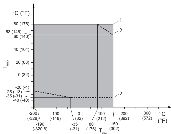
图 19: 允许的过程介质温度和环境温度，分离型
