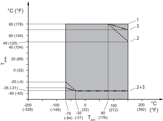
图 20: 允许的过程介质温度和环境温度，分离型（HS4 和 HS8 过程连接形式除外）
