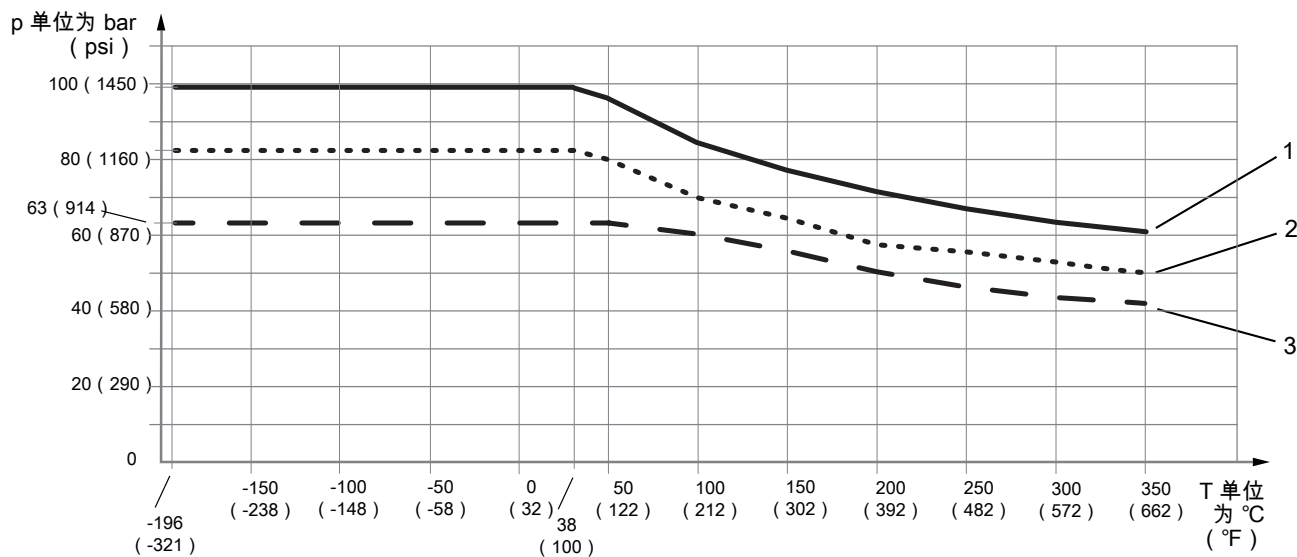
图 10: 与过程介质温度相关的允许过程压力
