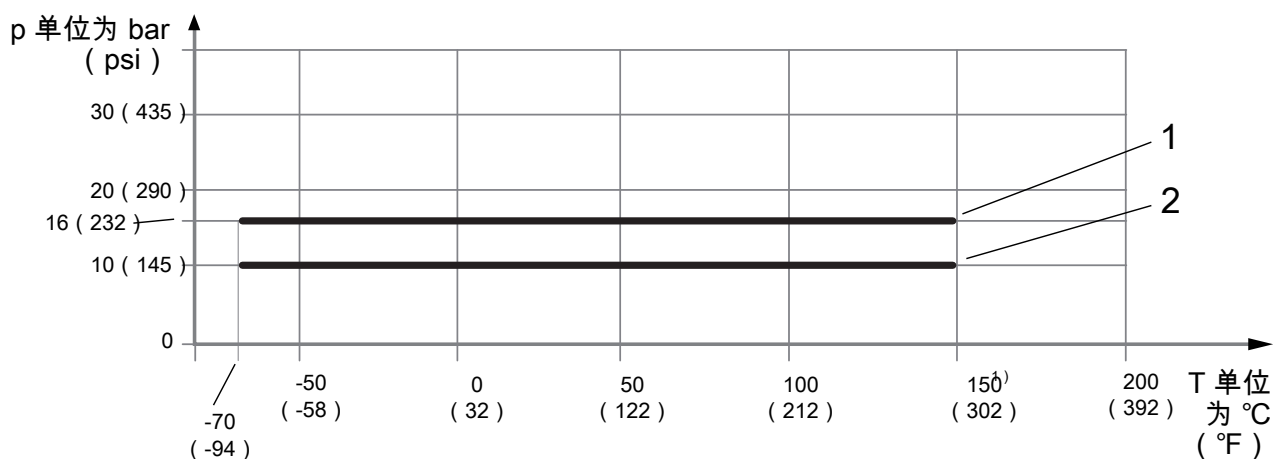
图 15: 与过程介质温度相关的允许过程压力
