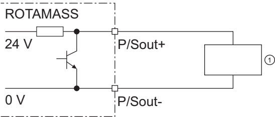
图 36: 配备内部上拉电阻的有源脉冲输出 P/Sout
