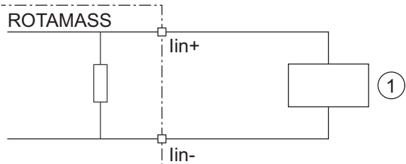
图 33: 外部设备与有源电流输出的连接
