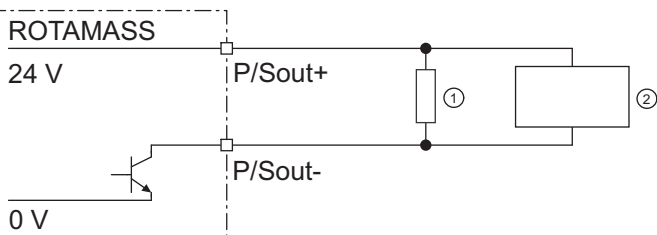
图 34: 有源脉冲输出连接 P/Sout
