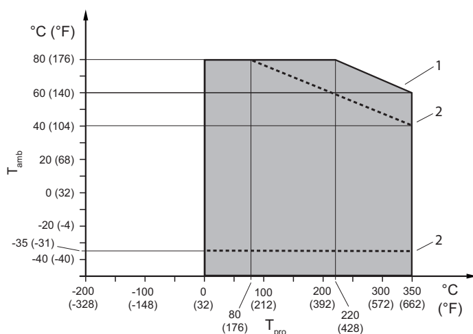
图 23: 允许的过程介质温度和环境温度，分离型
