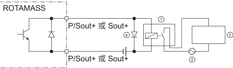
图 42: 适用于电磁阀电路的无源状态输出连接 P/Sout 或 Sout
