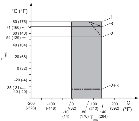
图 21: 允许的过程介质温度和环境温度，分离型，适用于 HS4 和 HS8 过程连接形式
