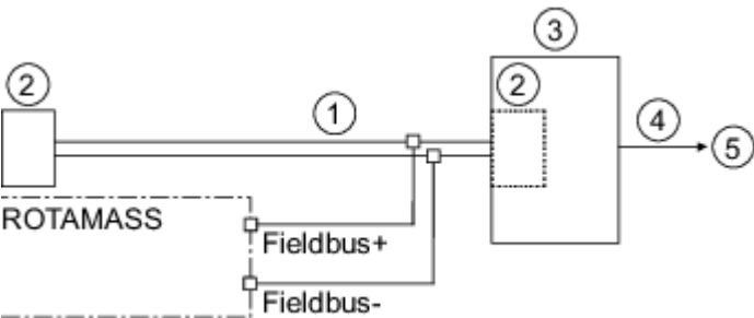
图 45: PROFIBUS PA 连接
