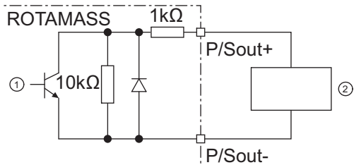
图 43: 配备开关放大器的无源脉冲或状态输出串联连接
