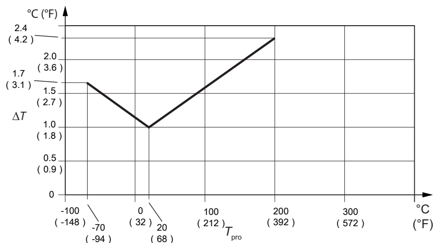
图 5: 温度精度
