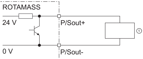
图 30: 配备内部上拉电阻的有源状态输出 P/Sout
