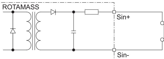
图 34: 状态输入连接
