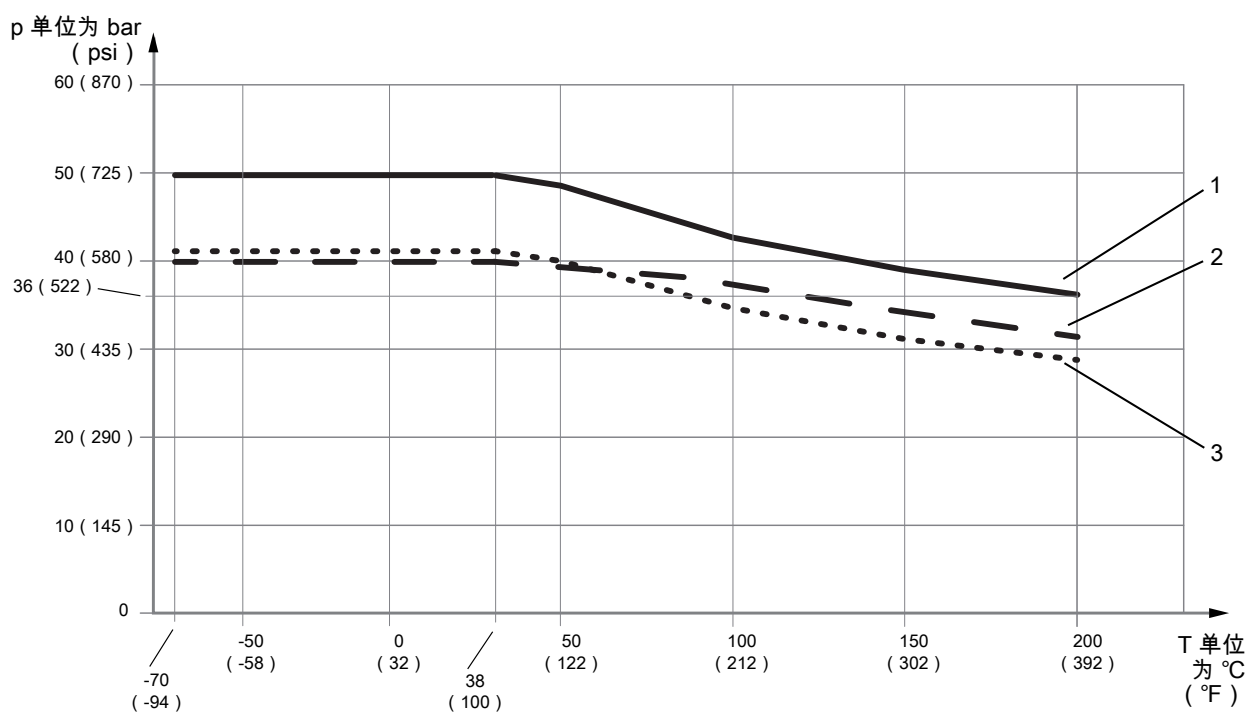
图 8: 与过程介质温度相关的允许过程压力
