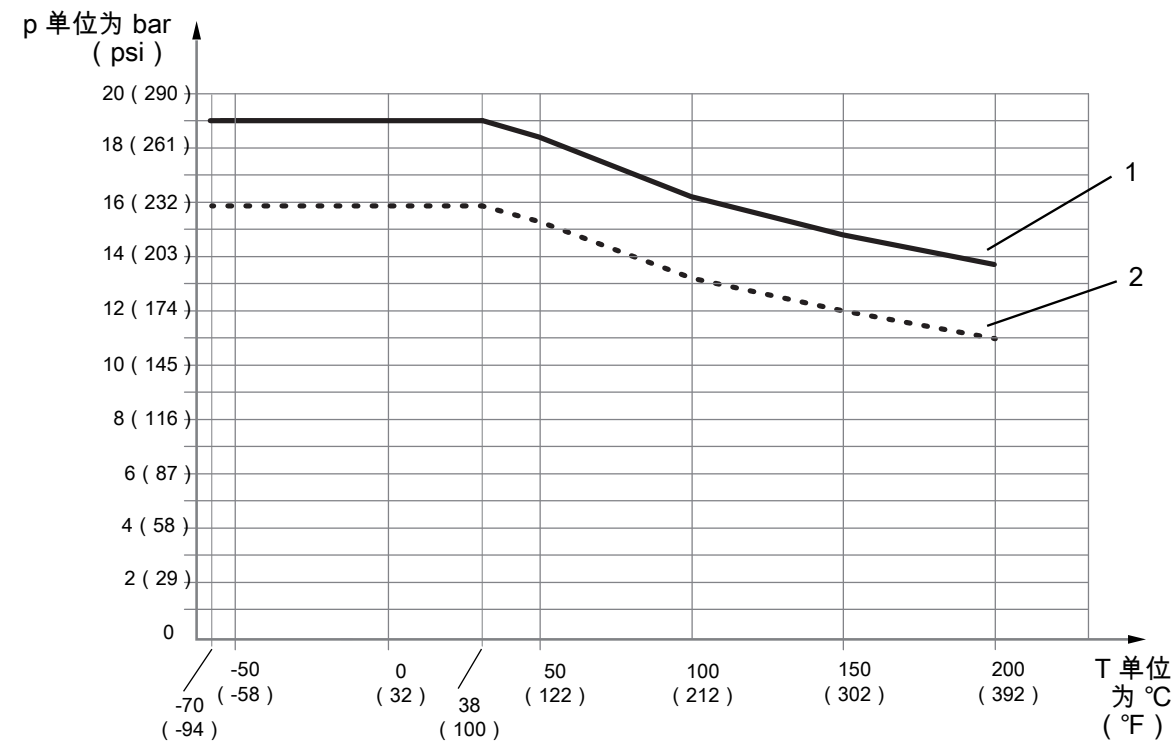
图 7: 与过程连接温度相关的允许过程压力
