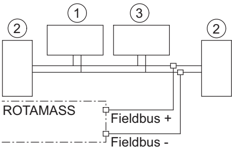
图 36: FOUNDATION 现场总线连接
