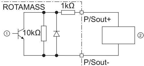
图 33: 配备开关放大器的无源脉冲或状态输出串联连接
