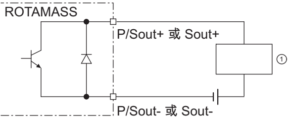
图 31: 无源状态输出连接 P/Sout 或 Sout
