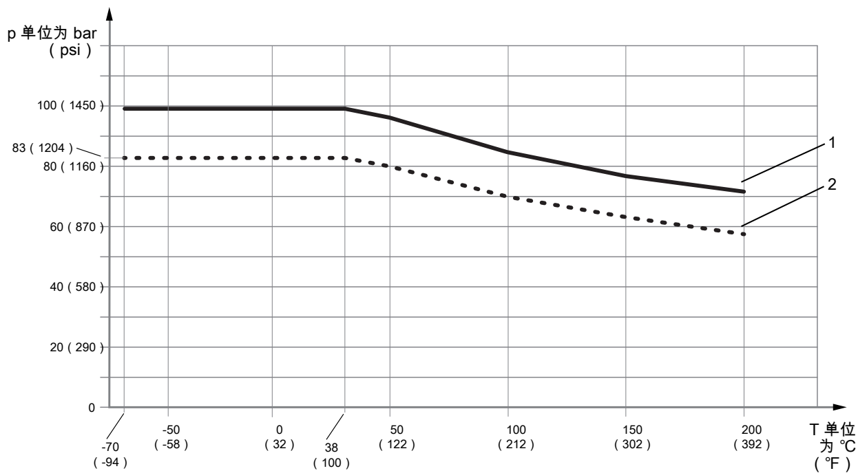
图 9: 与过程连接温度相关的允许过程压力
