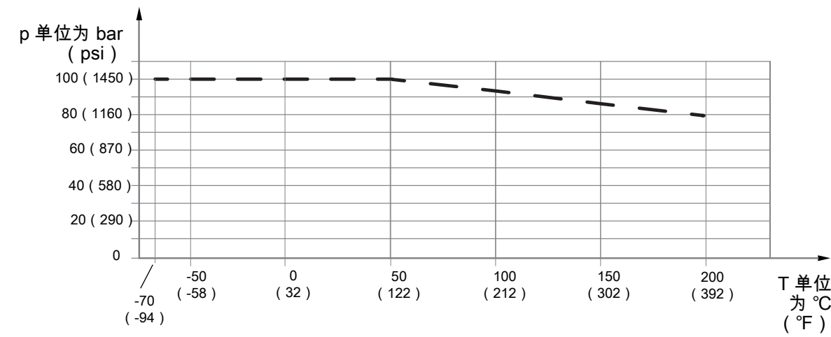
图 10: 与过程介质温度相关的允许过程压力，符合法兰 EN 1092-1 PN100
