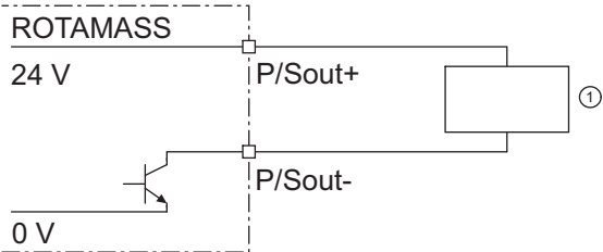
图 29: 有源状态输出连接 P/Sout
