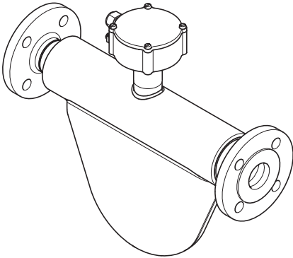
图 15: 带标准颈的分离型传感器
