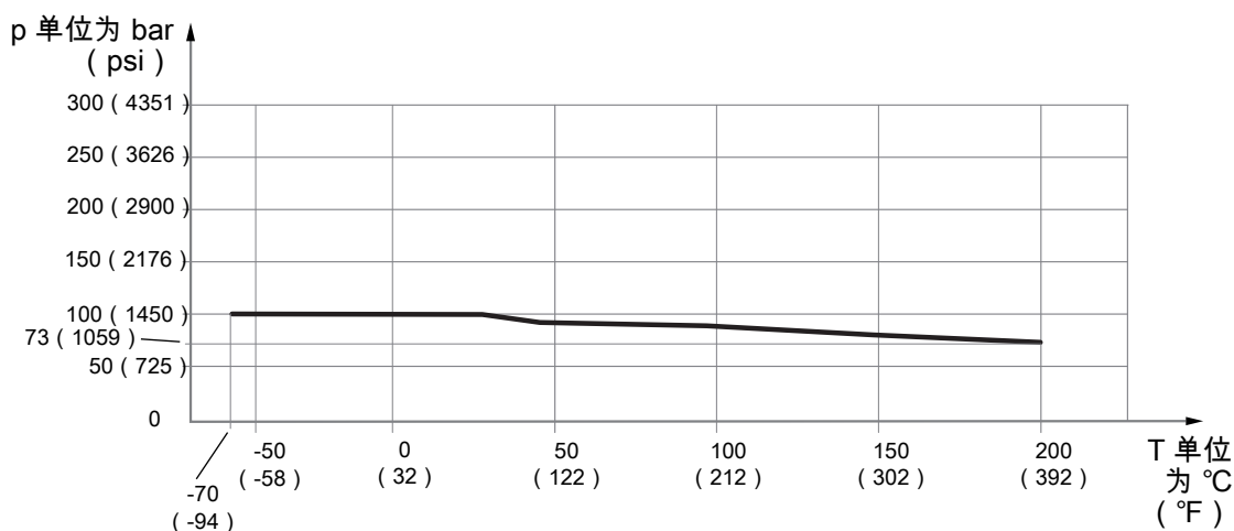
图 12: 与过程介质温度相关的允许过程压力
