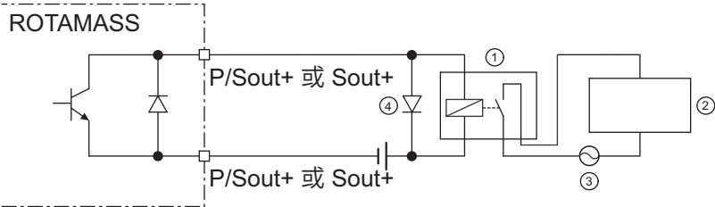
图 32: 适用于电磁阀电路的无源状态输出连接 P/Sout 或 Sout
