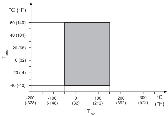
图 13: 允许的过程介质温度和环境温度，一体型
