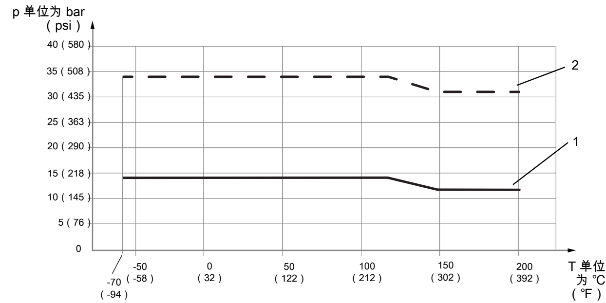
图 11: 与过程介质温度相关的允许过程压力
