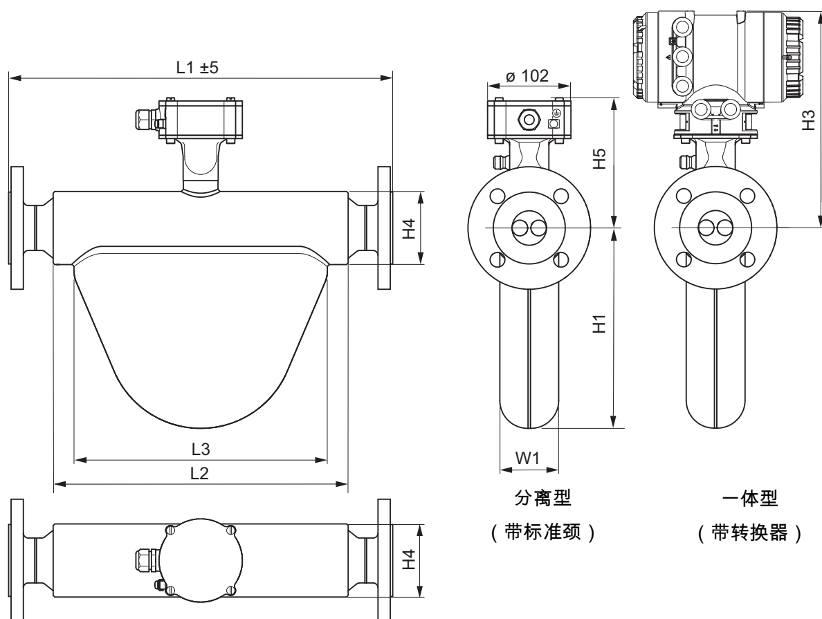
图 16: 尺寸 (毫米)
