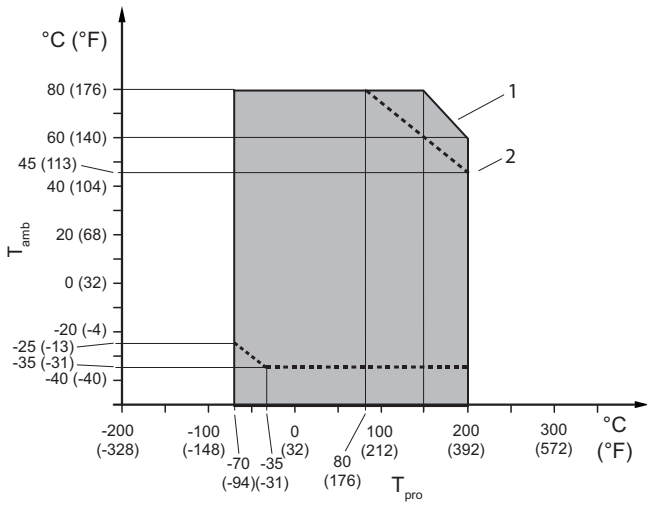
图 14: 允许的过程介质温度和环境温度，分离型
