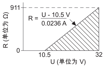
图 20: 最大负载电阻（根据外部供电电源电压）
