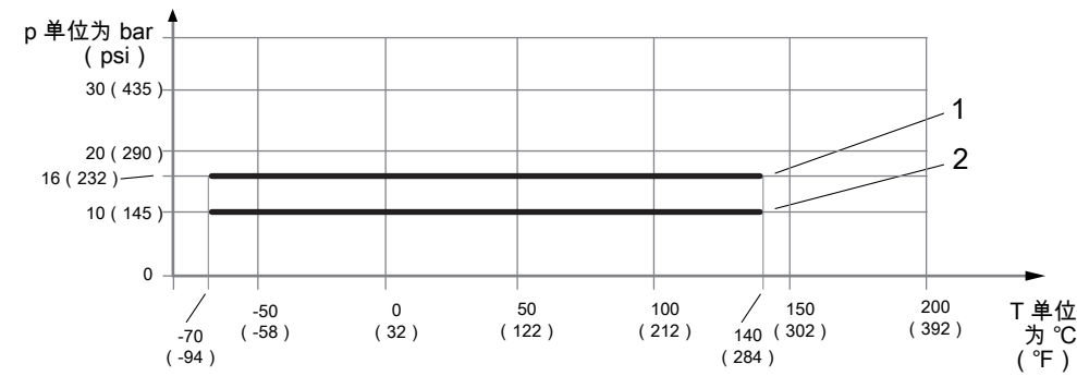
图 11: 与过程连接温度相关的允许过程压力
