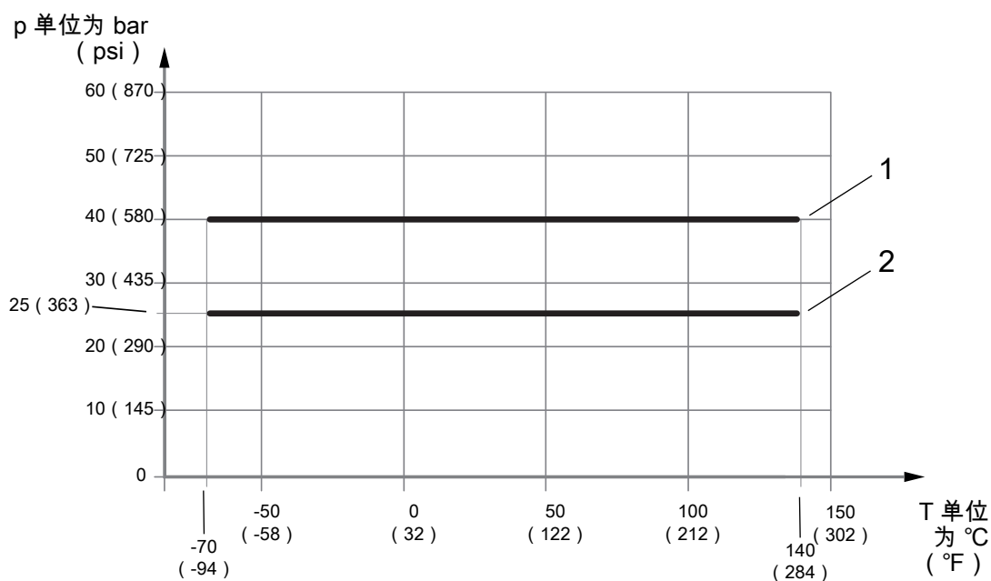
图 8: 与过程连接温度相关的允许过程压力
