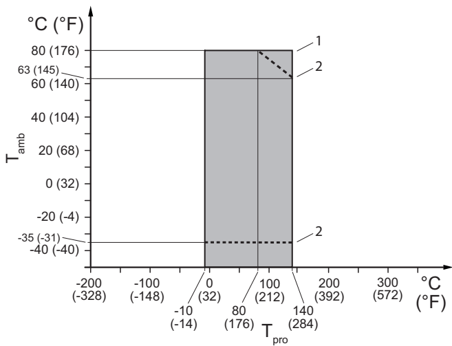
图 15: 允许的过程介质温度和环境温度，分离型，适用于 HS4 和 HS8 过程连接形式
