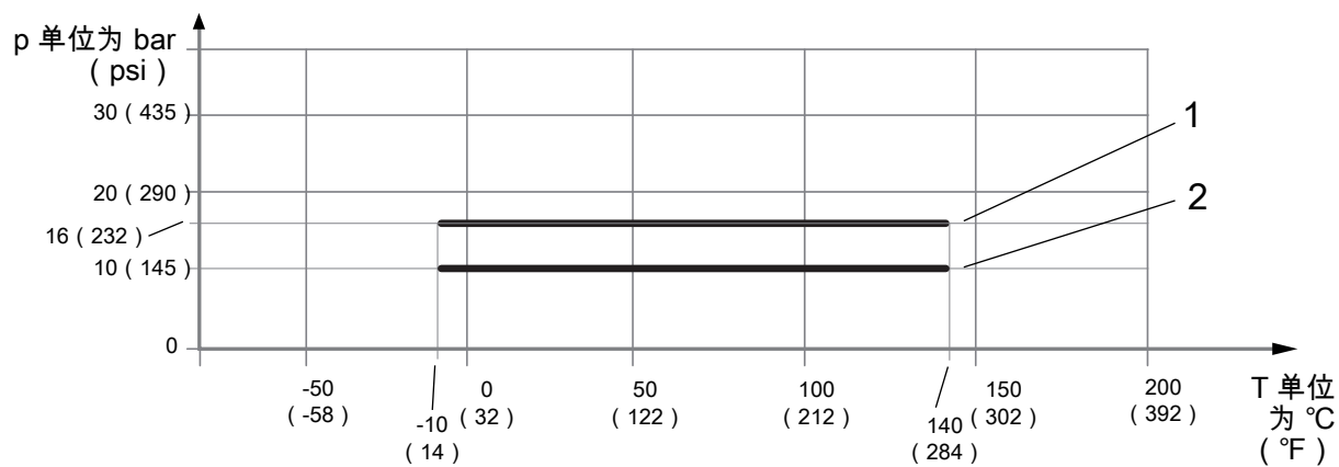
图 9: 与过程介质温度相关的允许过程压力
