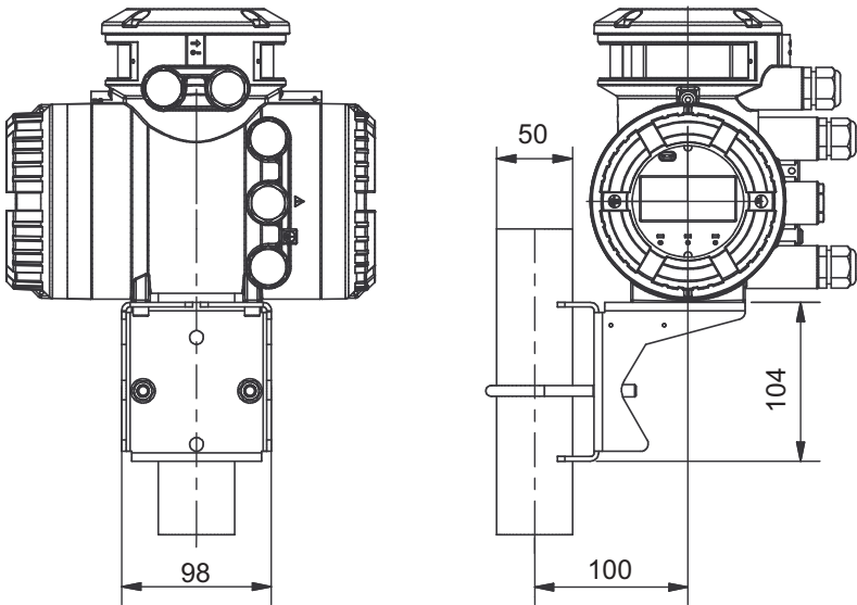
图 19: 转换器尺寸（单位：毫米），与安装托架连接
