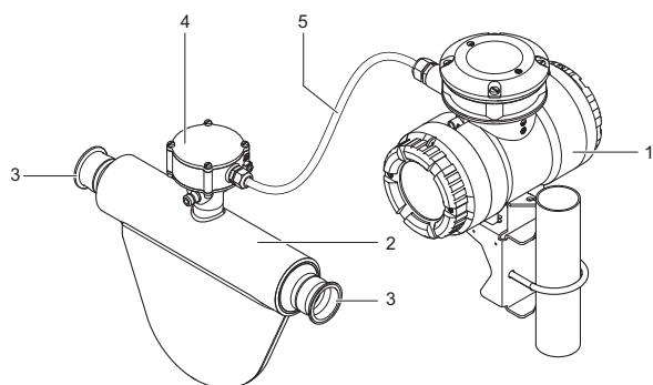
图 3: Rotamass 分离型流量计的配置
