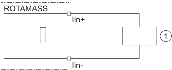
图 24: 外部设备与有源电流输出的连接
