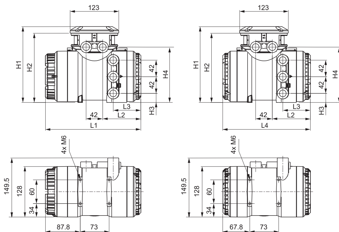
图 18: 转换器尺寸 (单位: 毫米) (左: 带显示器的转换器; 右: 不带显示器的转换器)
