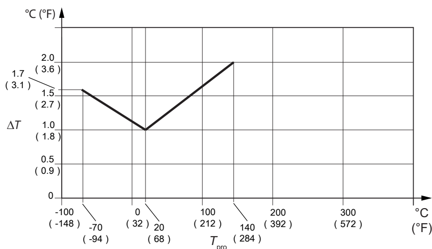
图 5: 温度精度展示
