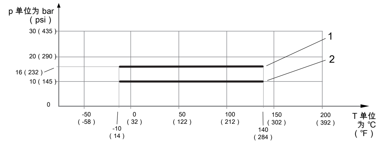
图 10: 与过程介质温度相关的允许过程压力
