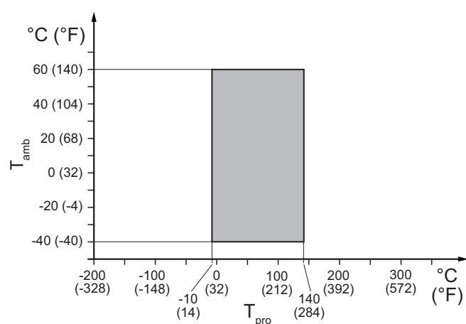
图 13: 允许的过程介质温度和环境温度，一体型，适用于 HS4 和 HS8 过程连接形式
