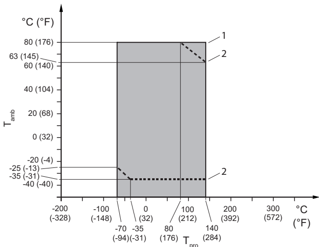
图 14: 允许的过程介质温度和环境温度，分离型，适用于 HS2 和 HS9 过程连接形式
