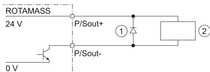
图 26: 配备机电计数器的有源脉冲输出 P/Sout 连接
