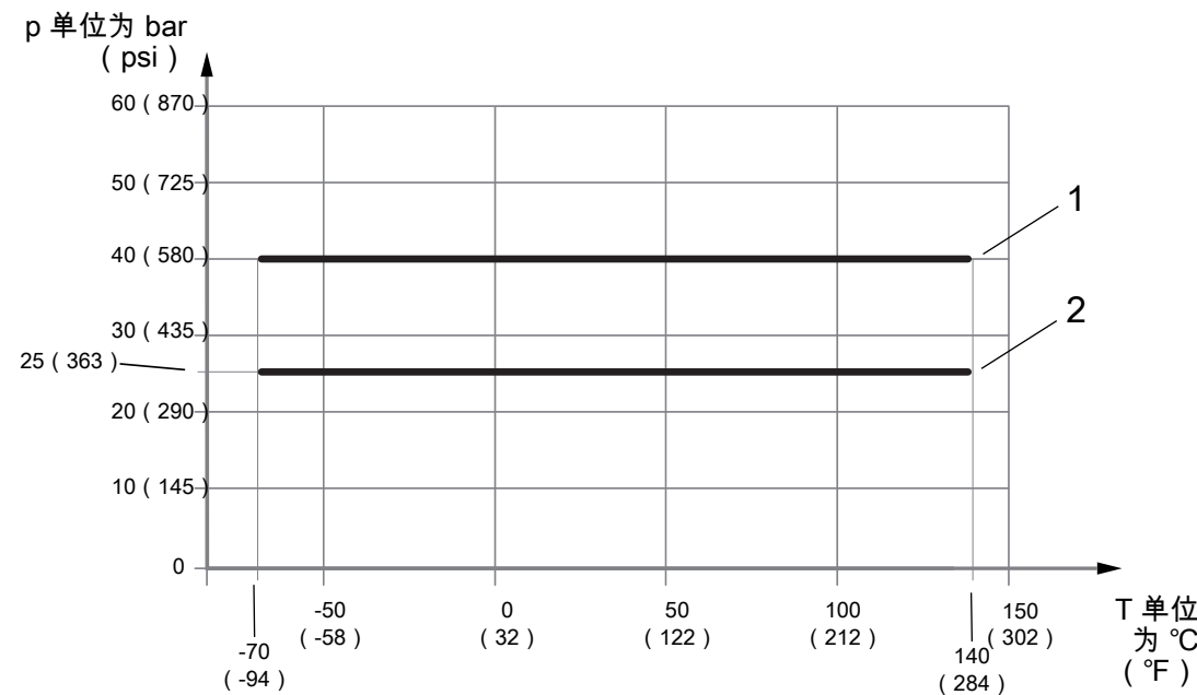
图 7: 与过程连接温度相关的允许过程压力
