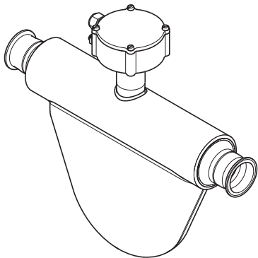
图 16: 带标准颈的分离型传感器
