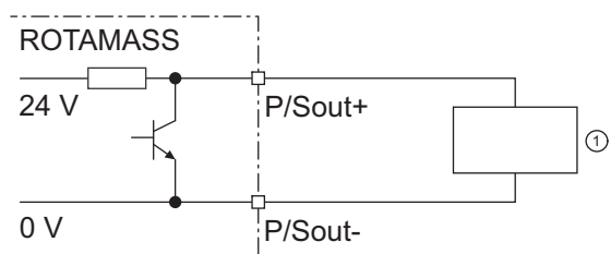
图 31: 配备内部上拉电阻的有源状态输出 P/Sout
