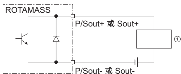
图 32: 无源状态输出连接 P/Sout 或 Sout
