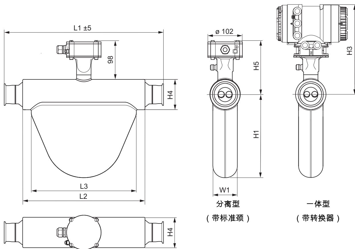
图 17: 尺寸 (毫米)
