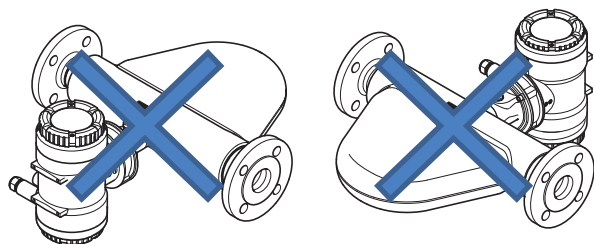
图 6: 需要避开的安装位置：流量计处于侧面位置
