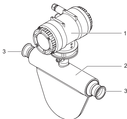
图 2: Rotamass 一体型流量计的配置
