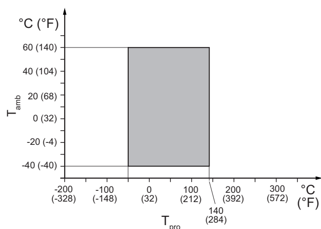
图 12: 允许的过程介质温度和环境温度，一体型，适用于 HS2 和 HS9 过程连接形式
