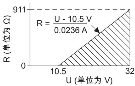
图 21: 最大负载电阻（根据外部供电电源电压）
