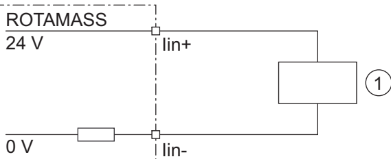
图 23: 外部设备与无源电流输出的连接
