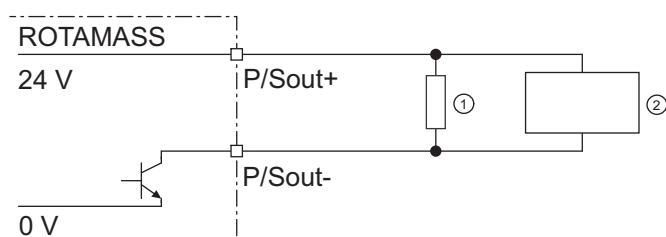
图 25: 有源脉冲输出连接 P/Sout
