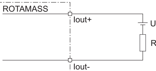
图 22: 无源电流输出连接 lout
