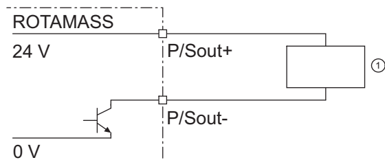
图 30: 有源状态输出连接 P/Sout
