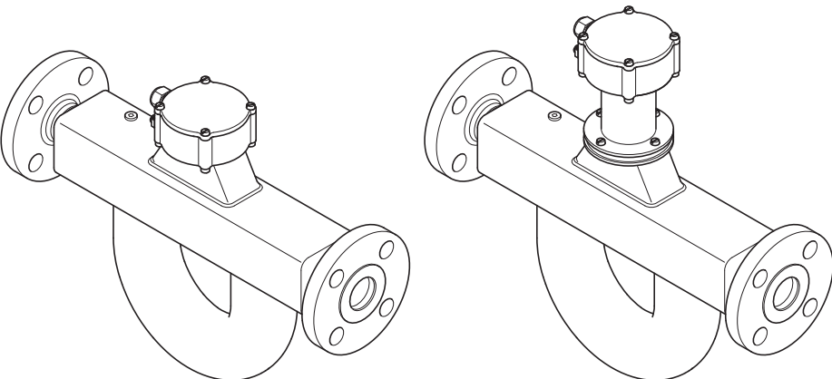
图 17: 带标准颈和加长颈的分离型传感器，适用于 34、36 和 38 仪表尺寸
