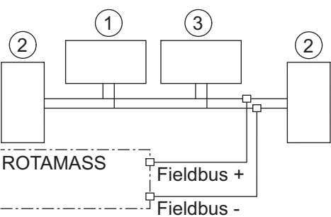
图 40: FOUNDATION 现场总线连接
