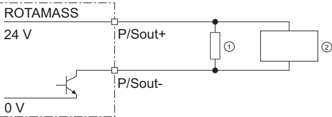
图 28: 有源脉冲输出连接 P/Sout
