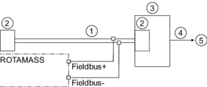
图 39: PROFIBUS PA 连接
