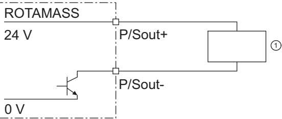
图 33: 有源状态输出连接 P/Sout
