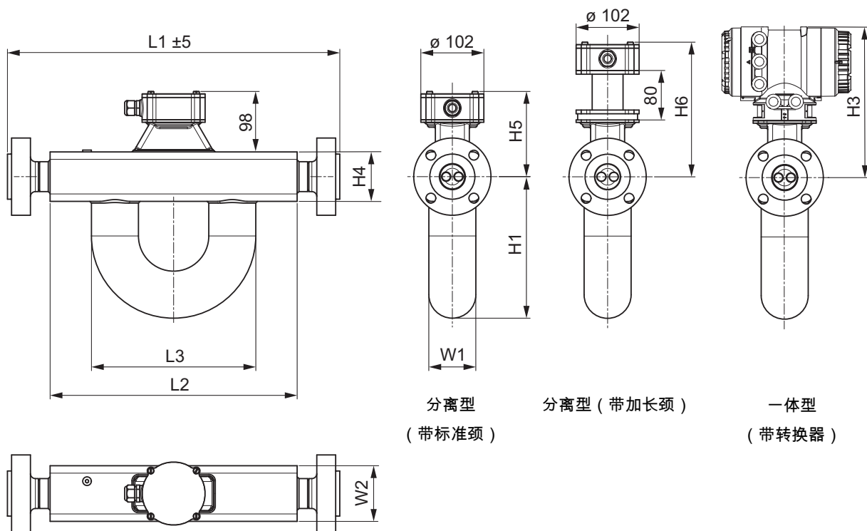
图 19: 尺寸 (毫米)
