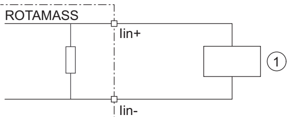
图 27: 外部设备与有源电流输出的连接
