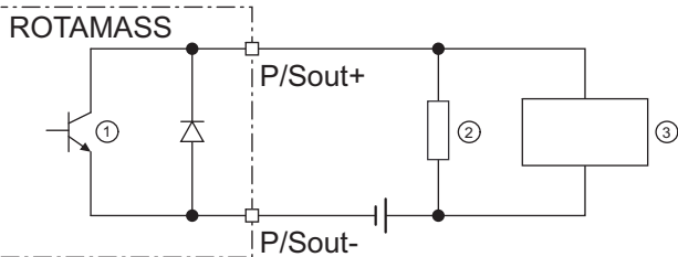
图 31: 配备电子计数器的无源脉冲输出 P/Sout 连接
