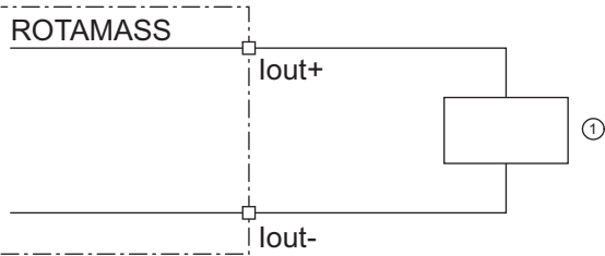
图 23: 有源电流输出连接 lout HART
