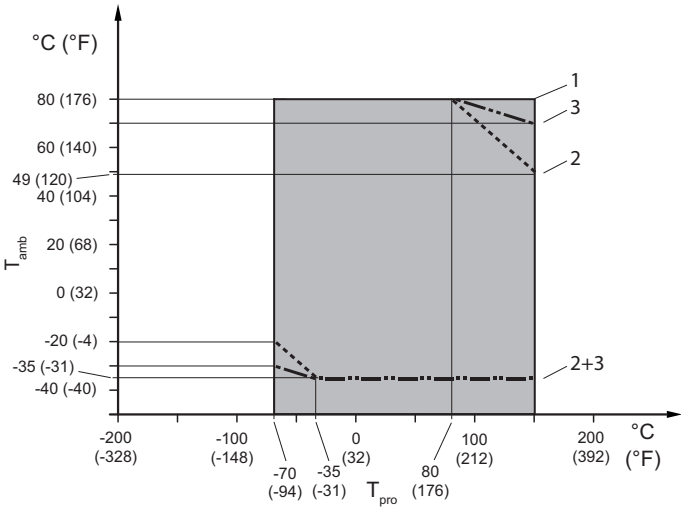
图 13: 允许的过程介质温度和环境温度，分离型
