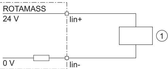
图 26: 外部设备与无源电流输出的连接
