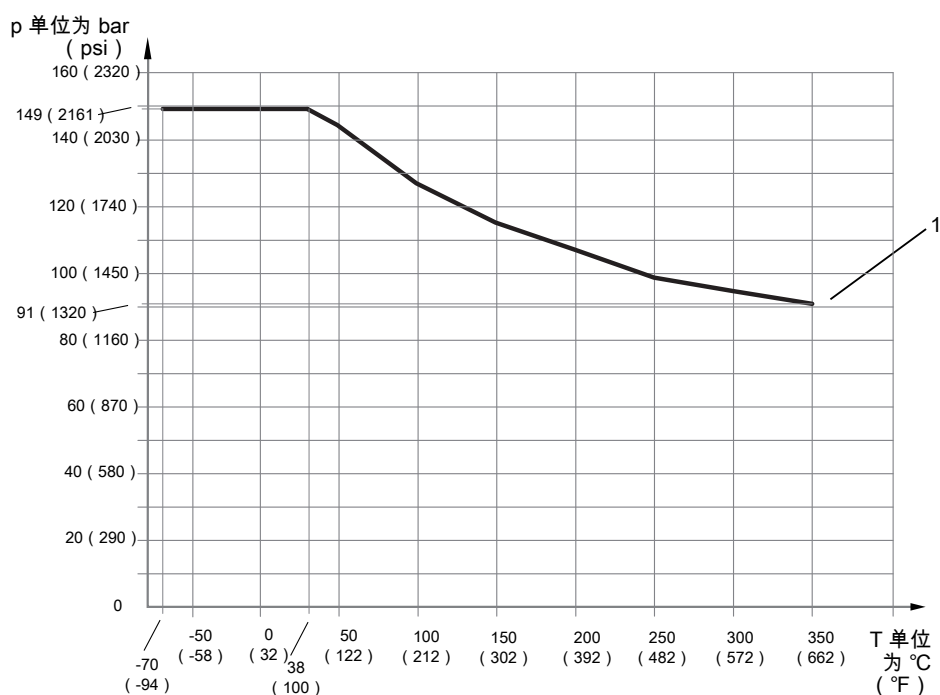
图 8: 与过程连接温度相关的允许过程压力
