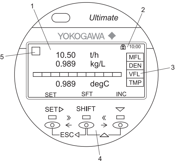
图 41: 显示器布局
