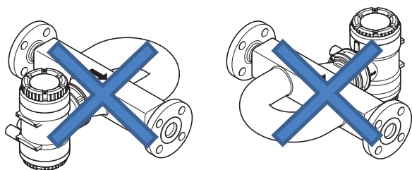
图 7：需要避开的安装位置：流量计处于侧面位置
