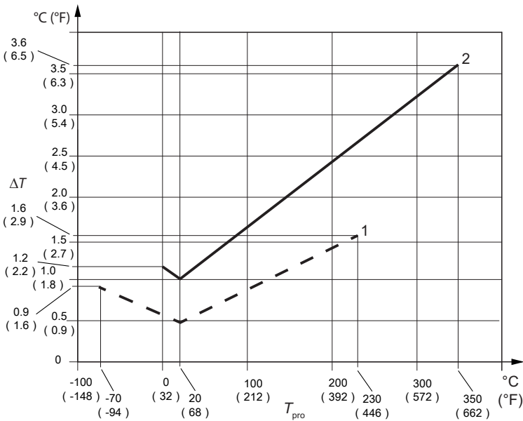
图 6: 温度精度
