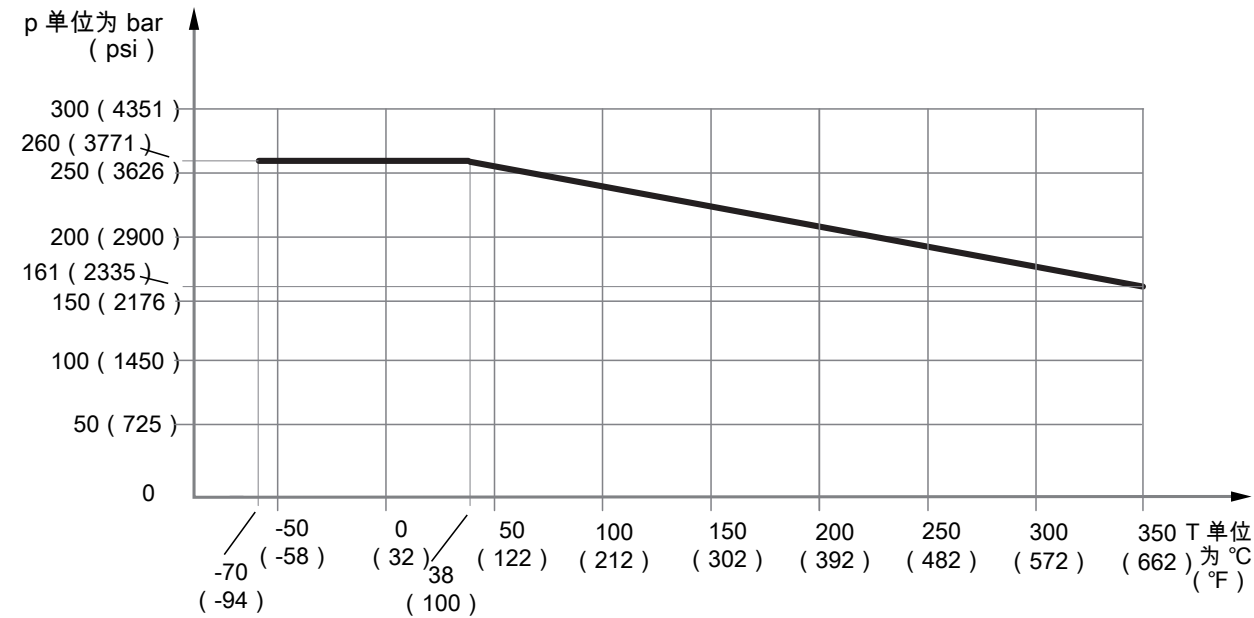
图 10: 与温度相关的允许过程压力
