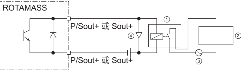
图 36: 适用于电磁阀电路的无源状态输出连接 P/Sout 或 Sout
