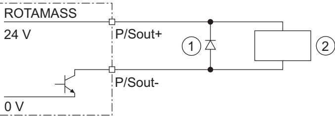
图 29: 配备机电计数器的有源脉冲输出 P/Sout 连接
