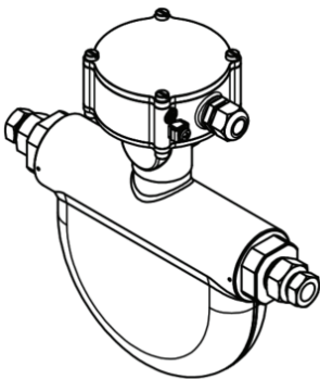
图 16: 带标准颈的分离型传感器，适用于 08 和 10 仪表尺寸
