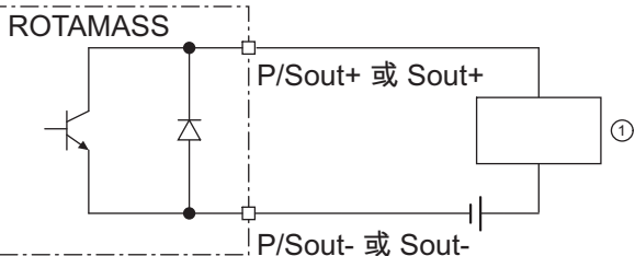
图 35: 无源状态输出连接 P/Sout 或 Sout
