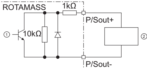
图 37: 配备开关放大器的无源脉冲或状态输出串联连接
