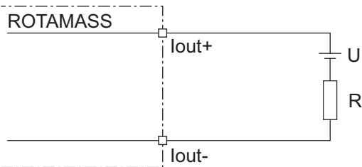
图 25: 无源电流输出连接 lout
