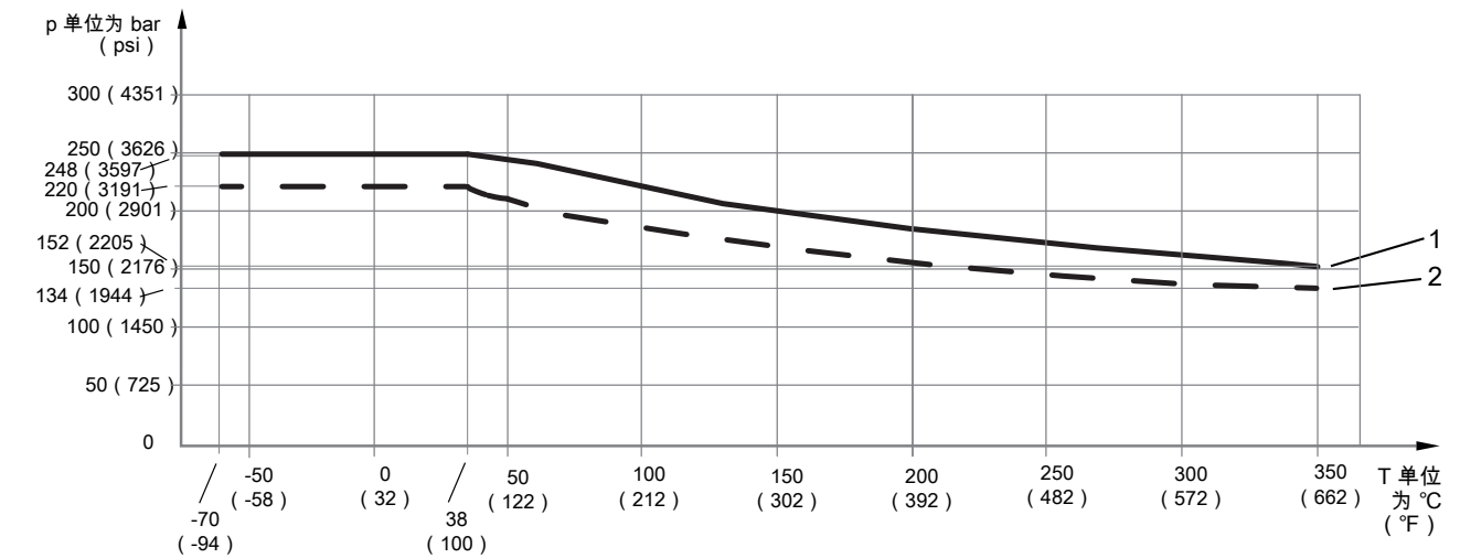
图 9: 与过程连接温度相关的允许过程压力
