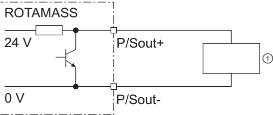
图 30: 配备内部上拉电阻的有源脉冲输出 P/Sout
