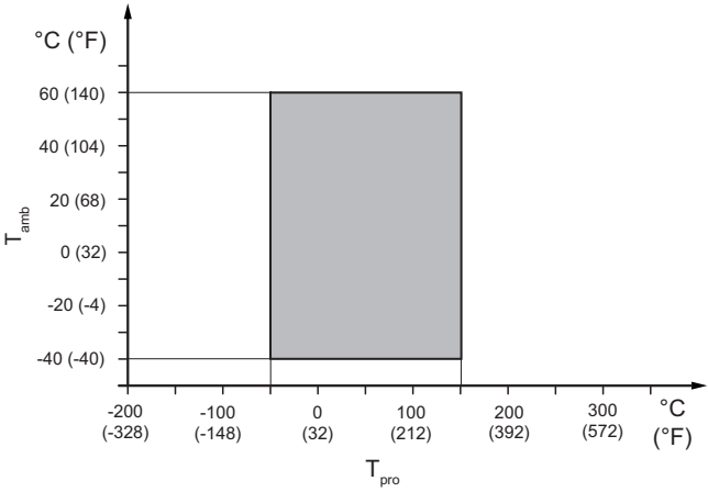
图 12: 允许的过程介质温度和环境温度，一体型
