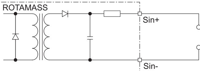
图 38: 状态输入连接
