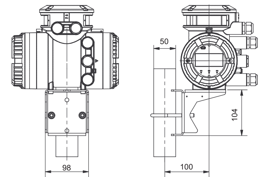
图 22: 转换器尺寸（单位：毫米），与安装托架连接
