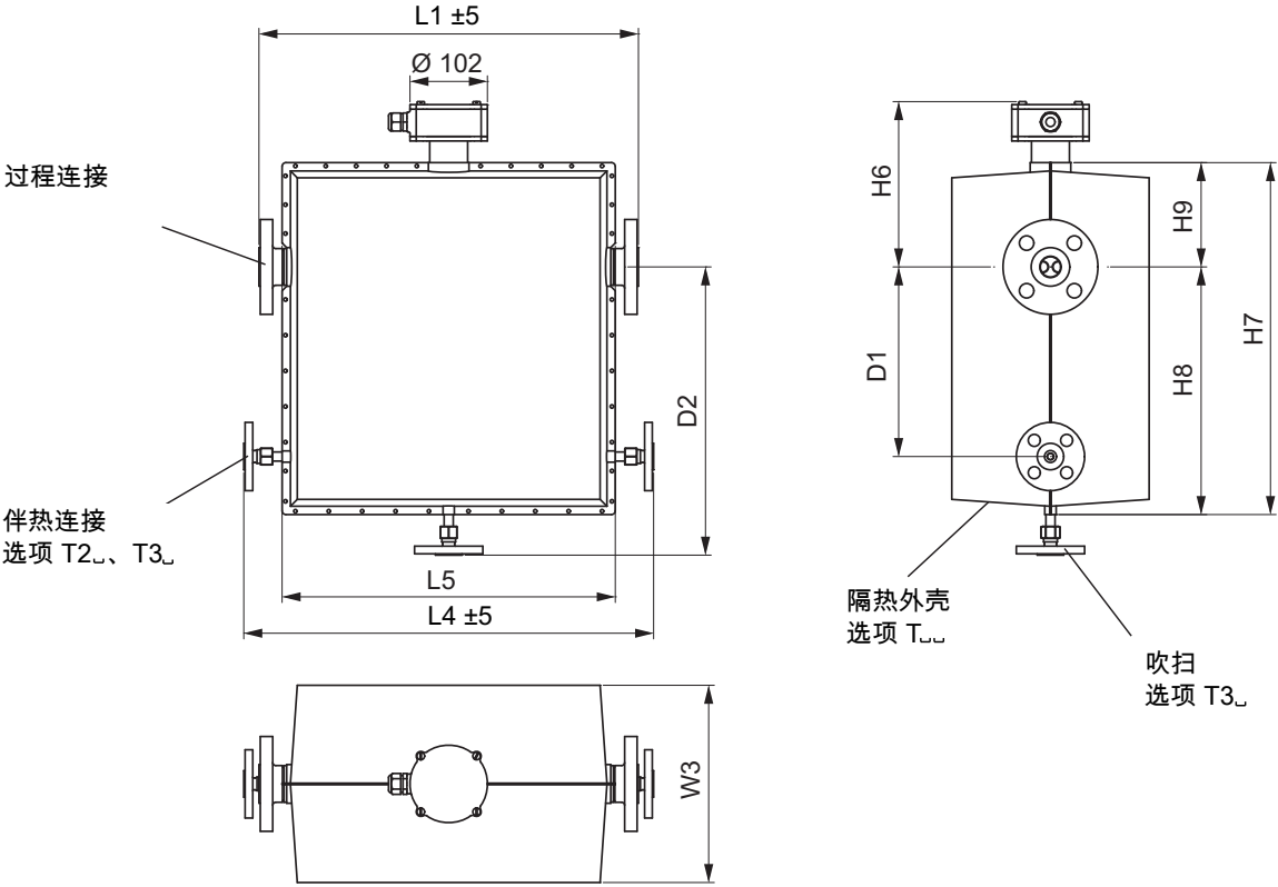
图 20: 尺寸 (毫米): 带隔热外壳的版本, 仅适用于 Intense 34、36 和 38 仪表尺寸
