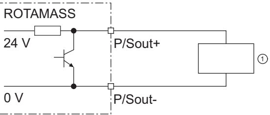
图 34: 配备内部上拉电阻的有源状态输出 P/Sout
