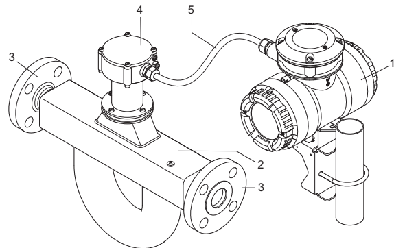
图 4: Rotamass 分离型流量计的配置 - 加长颈
