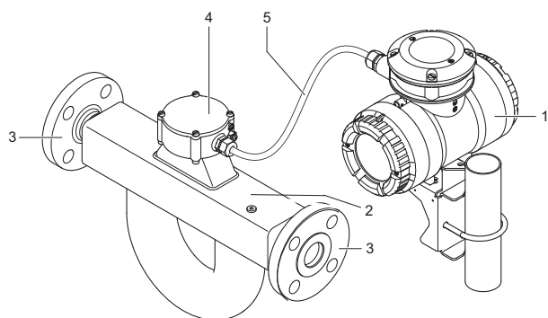
图 3: Rotamass 分离型流量计的配置
