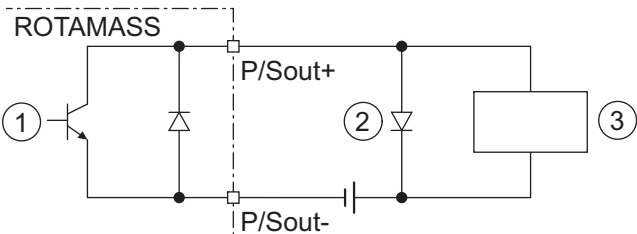
图 32: 配备机电计数器的无源脉冲输出 P/Sout 连接
